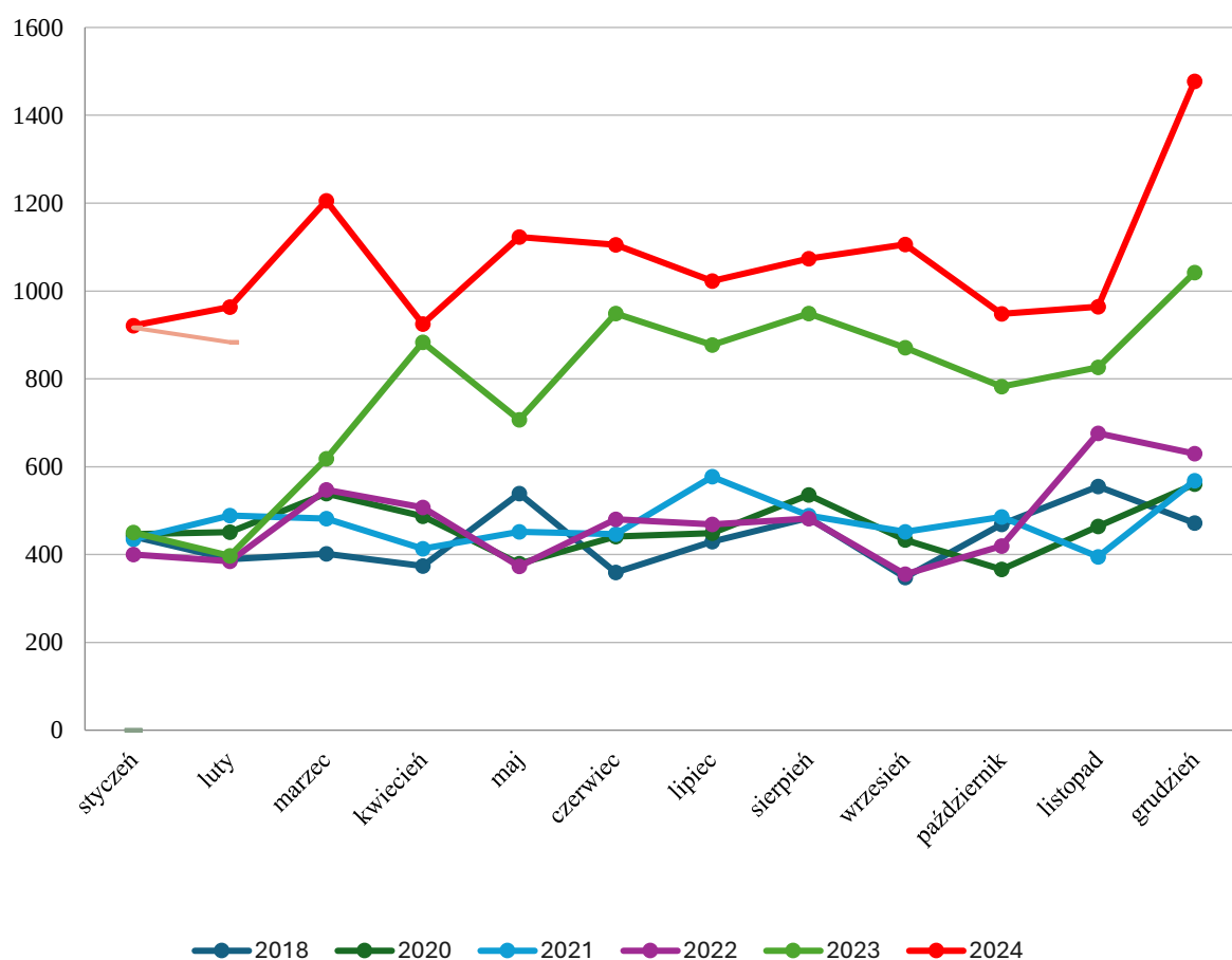
Ścieki dowożone na oczyszczalnię ścieków w latach 2018-2024 [m 3 ]
